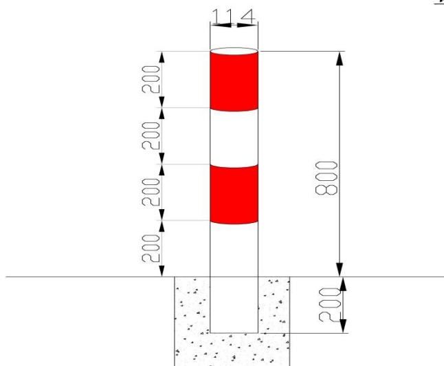
隔离柱尺寸图
